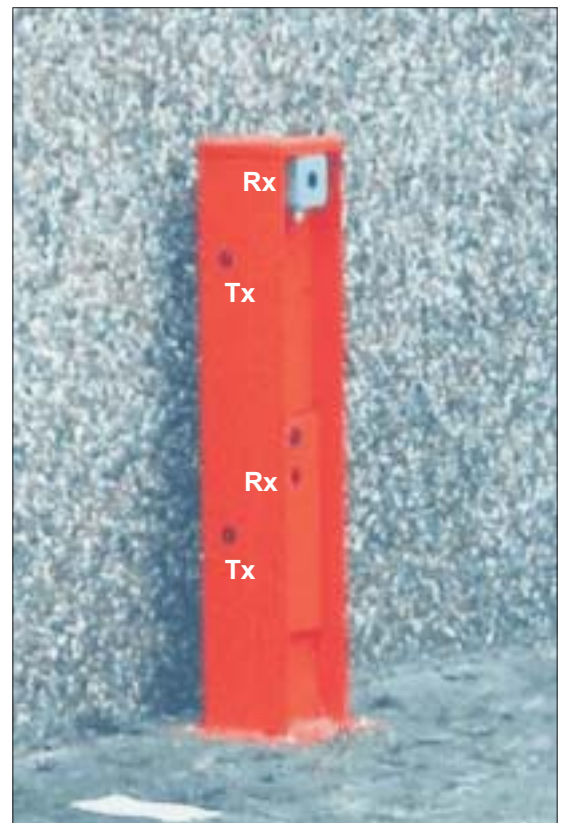
Versteckte Installation - Lichtschranken in einer Energieanschluss säule
