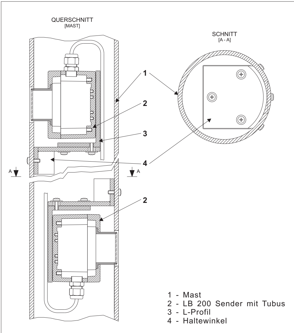
LB 200 - Einweglichtschanken im Mast montiert
